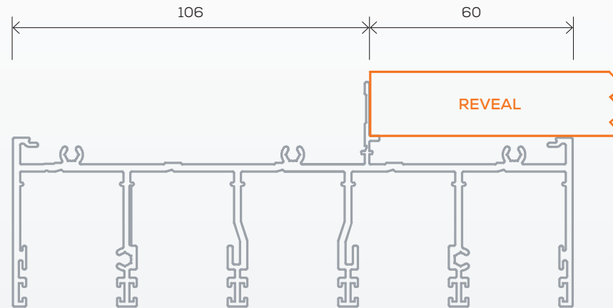
Signature Sliding Door (166mm)
