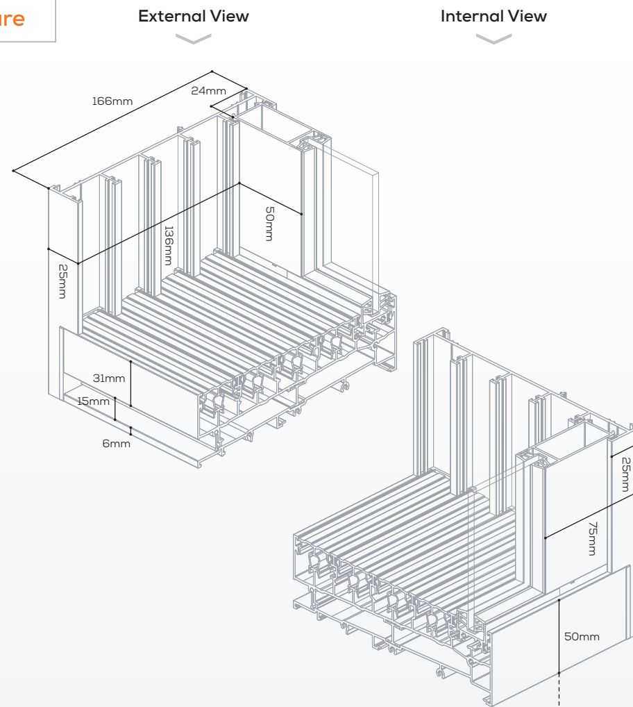
Signature Sliding Door (166mm)
